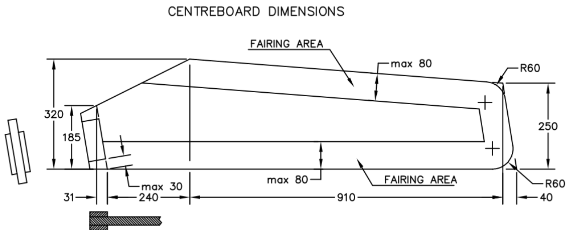
E.3.3.1. CENTREBOARD DIAGRAM
